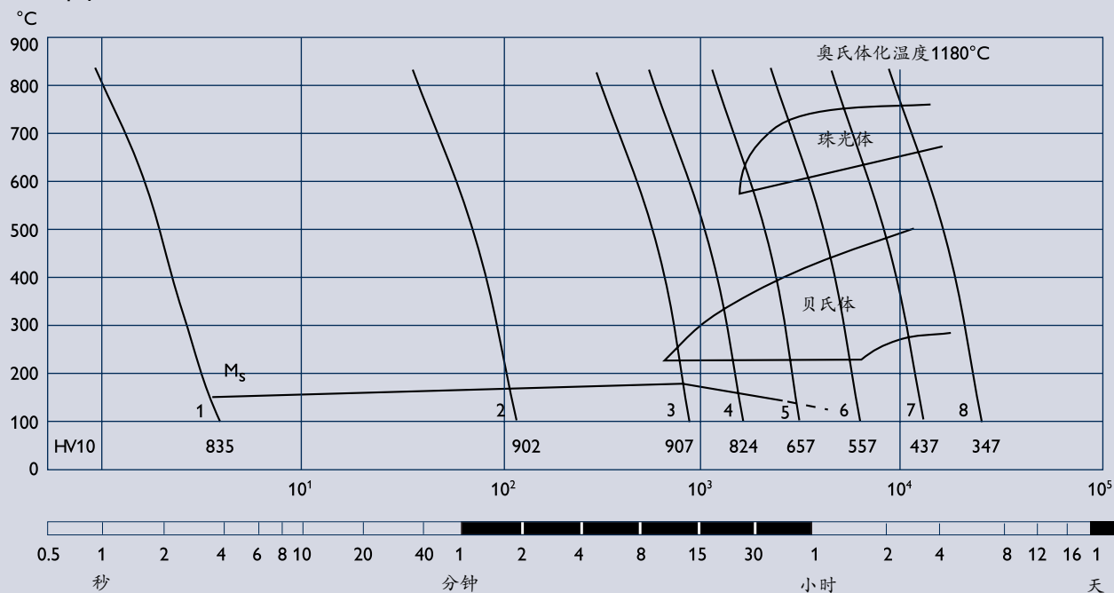
CCT 图
