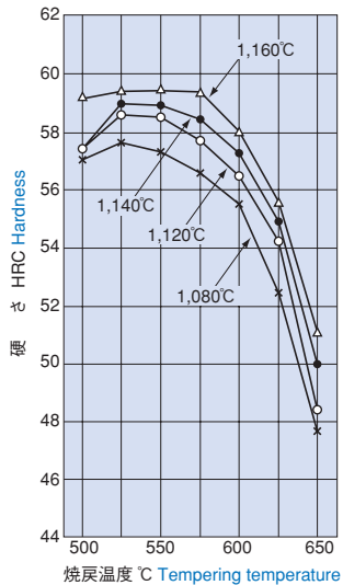
YXR33の焼入れ、焼戻し硬さ曲線 YXR33 Tempered hardness
