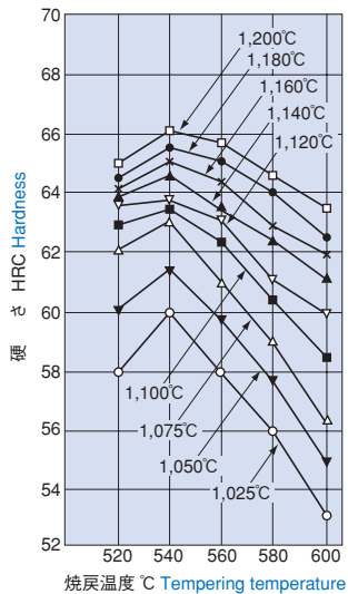
HAP10の焼入れ、焼戻し硬さ曲線 HAP10 Tempered hardness
